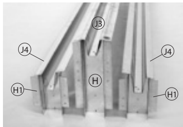
Nur Gr. 5 u. 7 / Sizes 5 and 7 only Taille 5 + 7 / Misura 5 + 7 Dachträger (J4) und Firststütze (H1) Roof beams (J4) and ridge supports (H1) porte-toit (J4) et support de faitière (H1) trave tetto (J4) sostegno colmo (H1)
